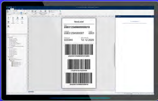
Designer-Schnittstelle
