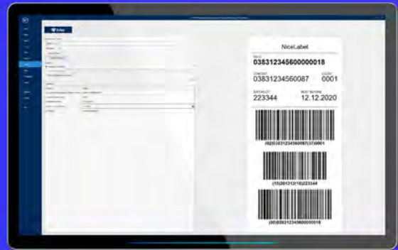
Druckbediener-Schnittstelle
